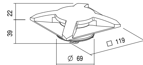
BIA MAXI SQUARE FOUR EM
