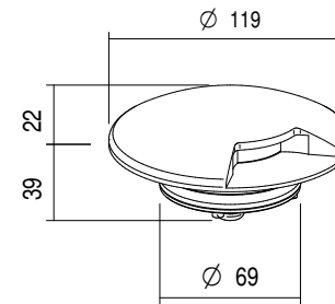
BIA MAXI ROUND SINGLE EM
