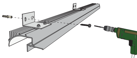
Installation with fixing brackets Installazione tramite staffe di fissaggio
